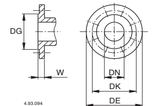
Flanges EN 1092-2
